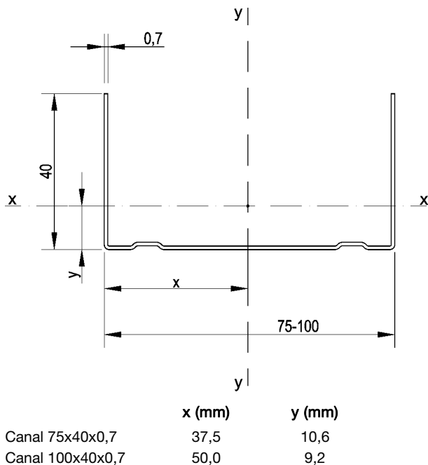
Figura 2.2: Canal exterior tipo.
