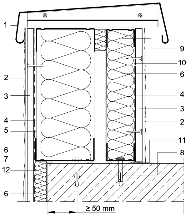
Figura 6.10: Coronación W388 (W387).
