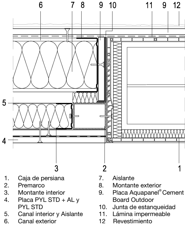
Figura 6.9: Encuentro con jamba y persiana W388 (W387).
