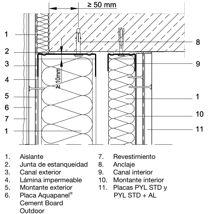
Figura 6.11: Encuentro con forjado W388 (W387).
