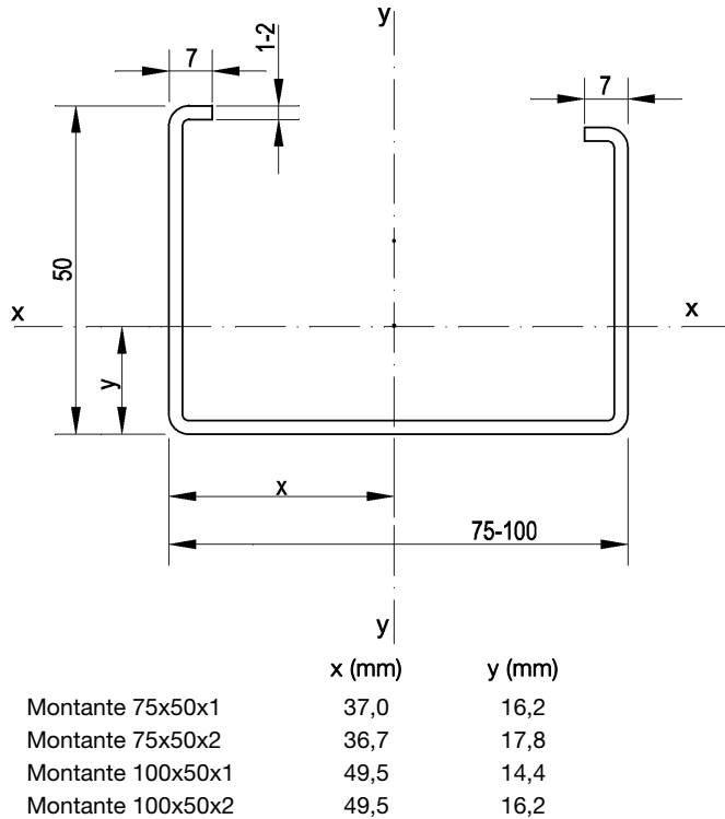
Figura 2.1: Montante exterior tipo.
