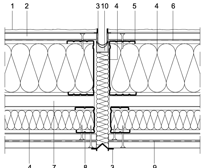
Figura 6.4: Junta de control superficial del sistema Aquapanel® Outdoor W388 (W387).
