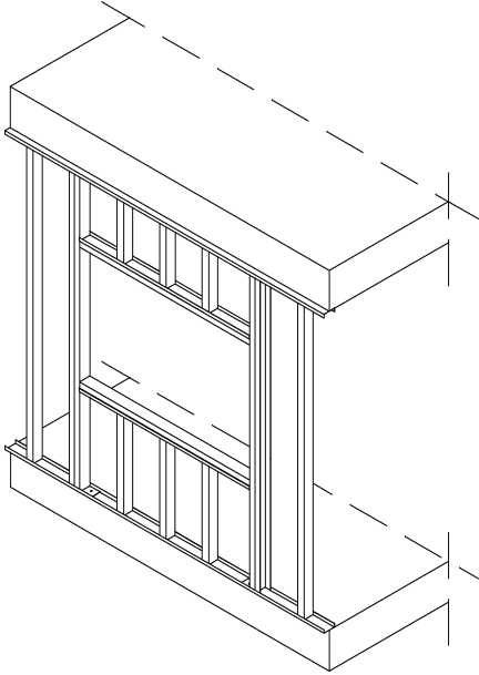
Figura 6.9: Vista del montaje de la subestructura metálica.
