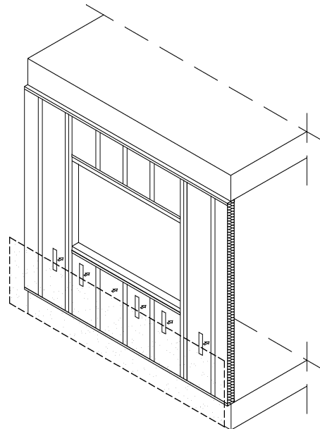
Figura 6.10: Vista del montaje del aislante.
