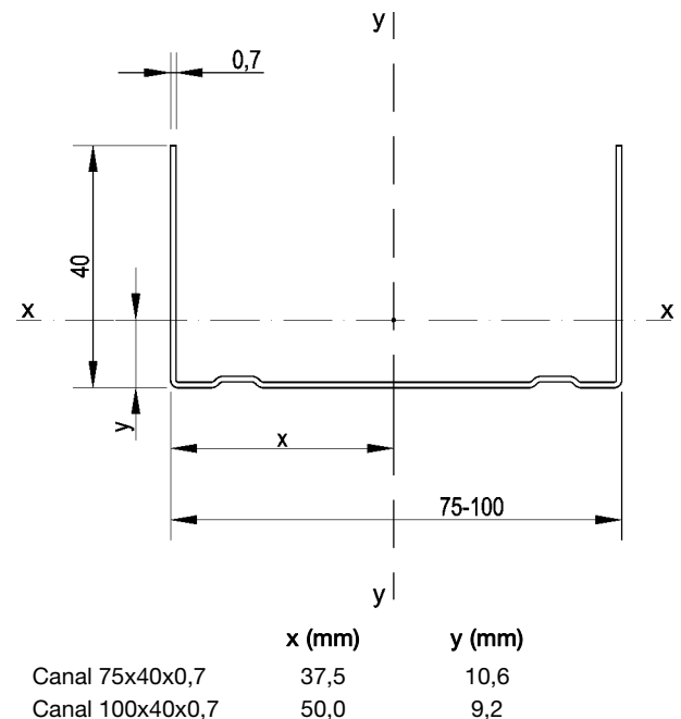
Figura 2.2: Canal tipo.
