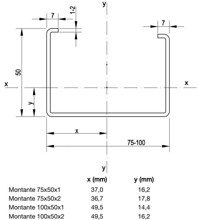
Figura 2.1: Montante tipo.
