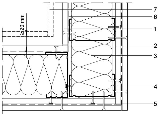
Figura 6.6: Esquina saliente del sistema Aquapanel® Outdoor W384.
