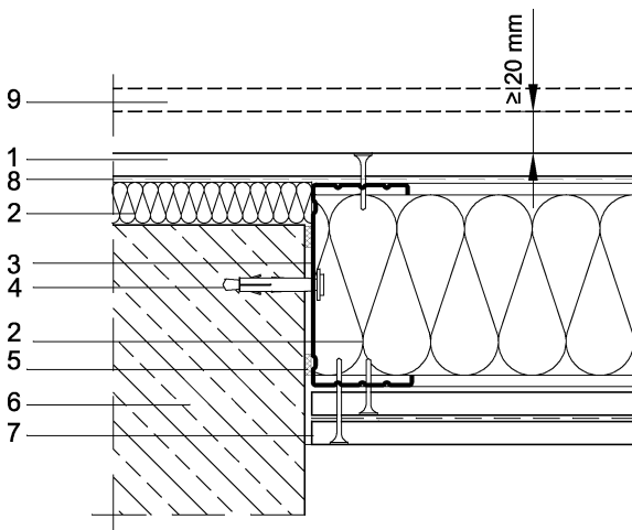
Figura 6.2: Sección horizontal del sistema Aquapanel® Outdoor W384.
